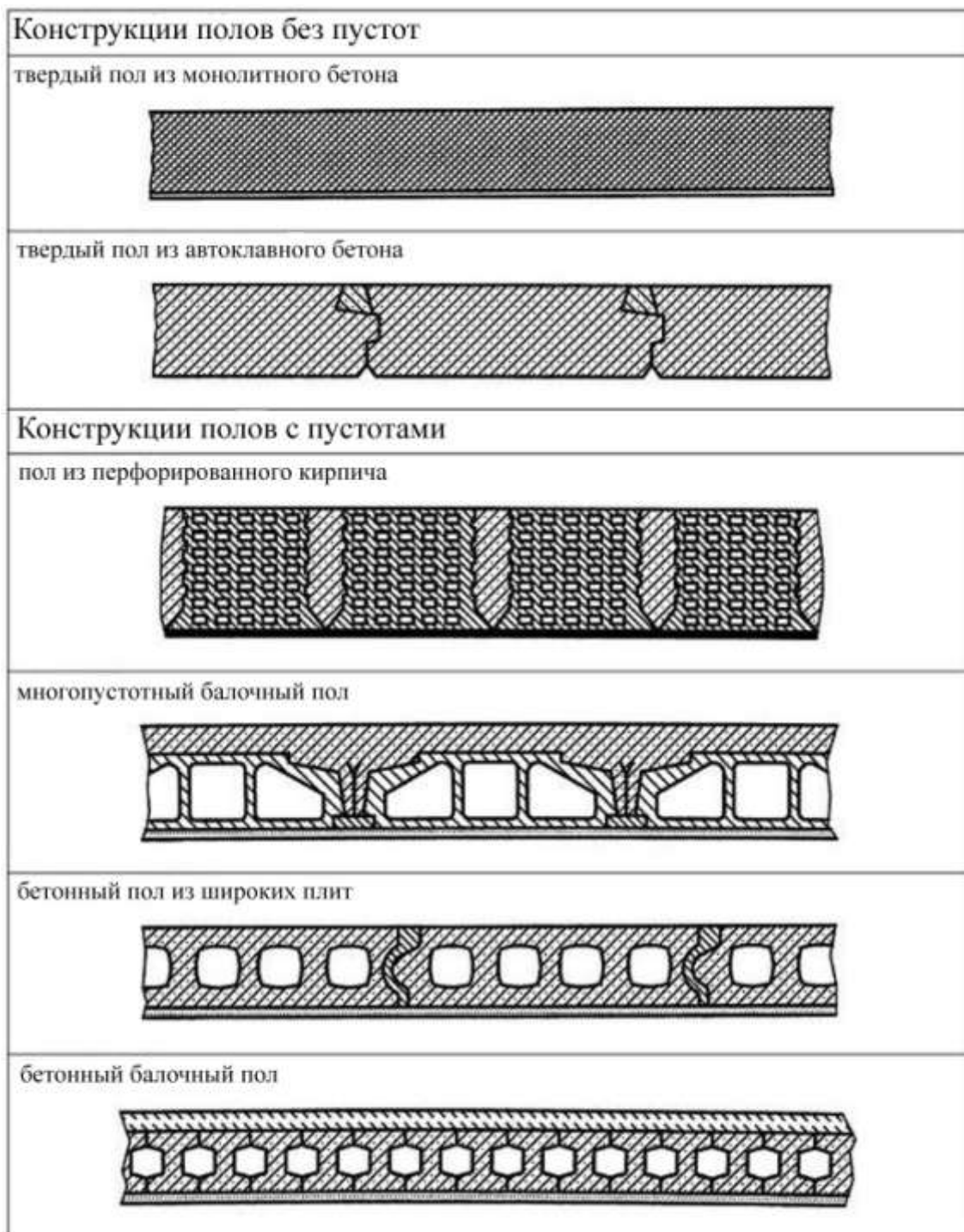
Рисунок В.1 – Основные типы однородных конструкций пола
