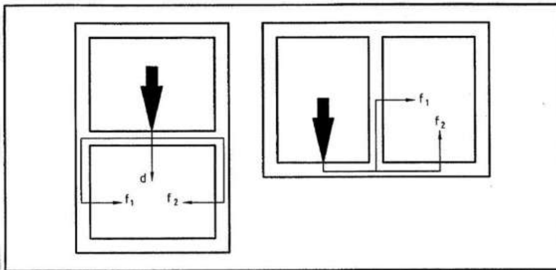
Рисунок 1 – Определение путей звукопередачи между двумя помещениями, расположенными один над другим и рядом друг с другом *
